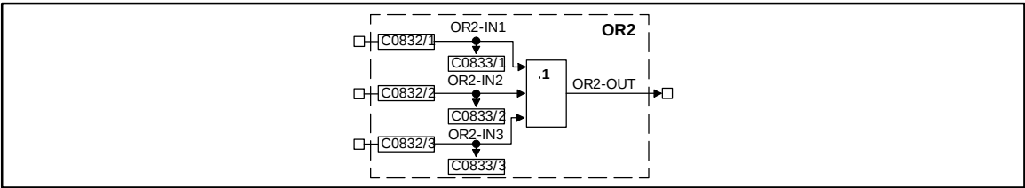
Fig. 7-130 Logic OR (OR2)
