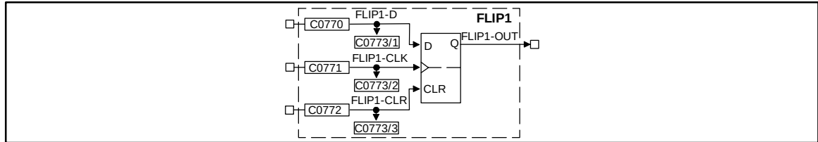
Flipflop (FLIP1)
